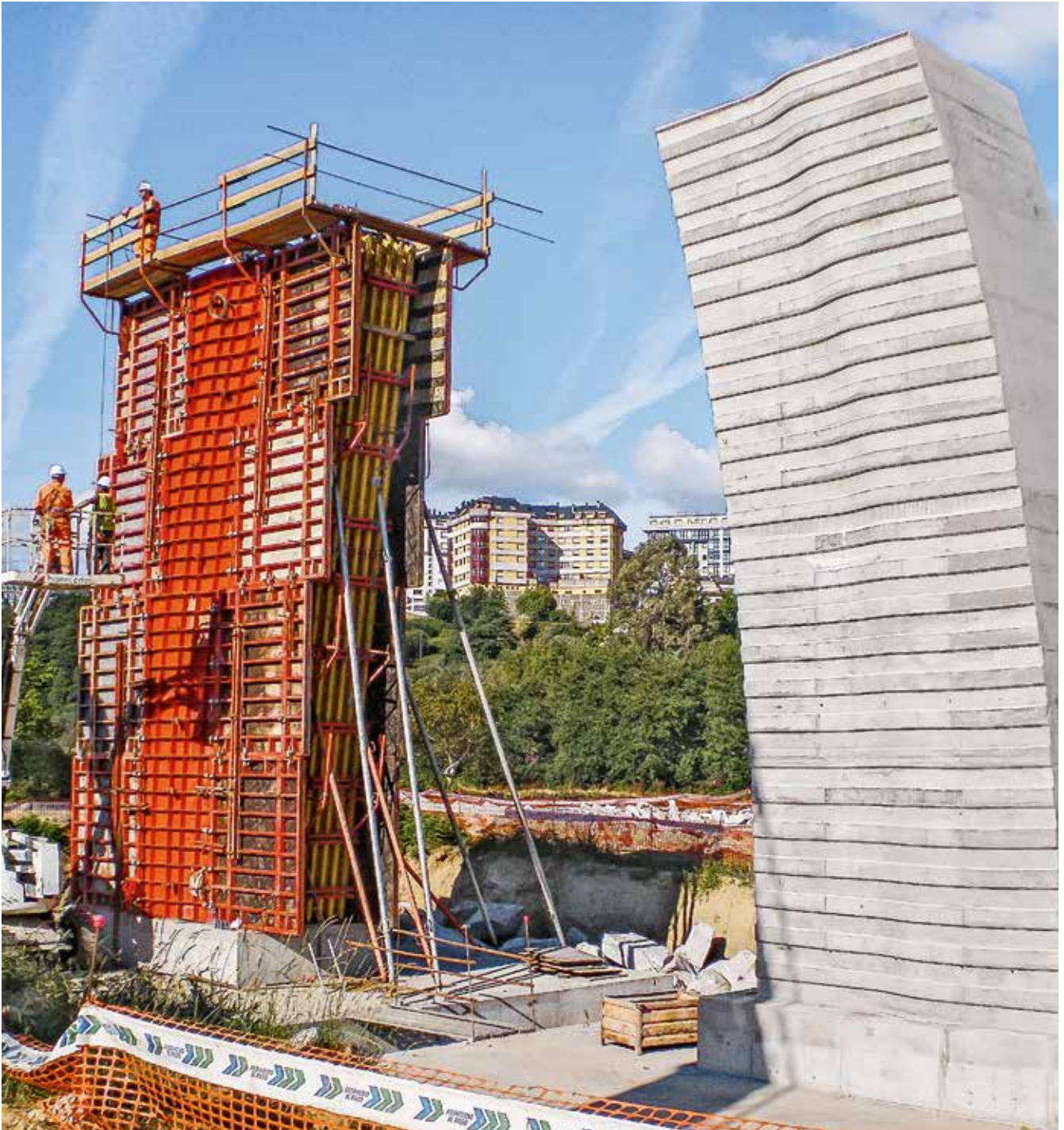
교각에 사용된 TRIO : 추가 나무 문양으로 흥미로운 표면 구조가 됩니다.
