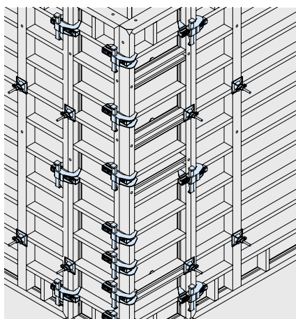
높이 3.30 m까지는 앵커 2개만으로 가능하며, BFD 얼라인먼트 커플러는 3개면 패널 조인트에 충분합니다.
