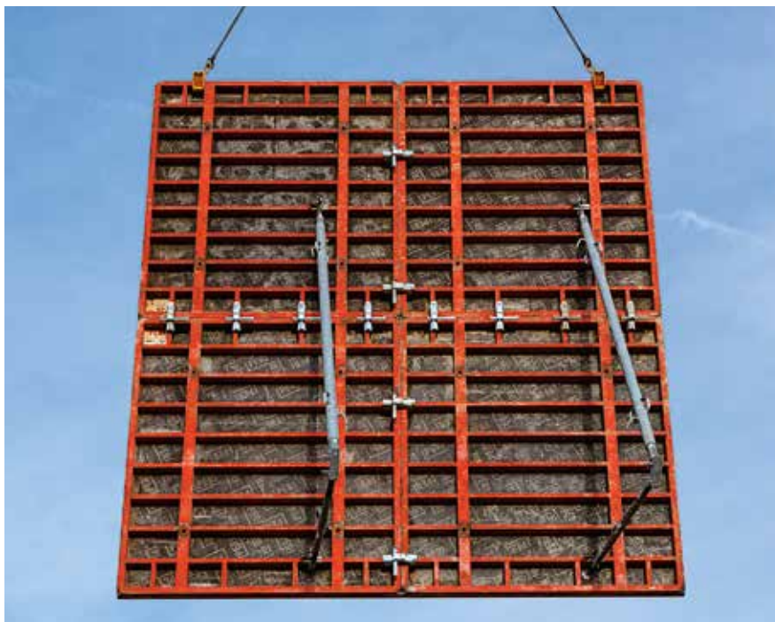
최대 5.40 m 높이 연장의 경우, 원형 보강대로 인해 단 하나의 BFD 얼라인먼트 커플러면 충분합니다
