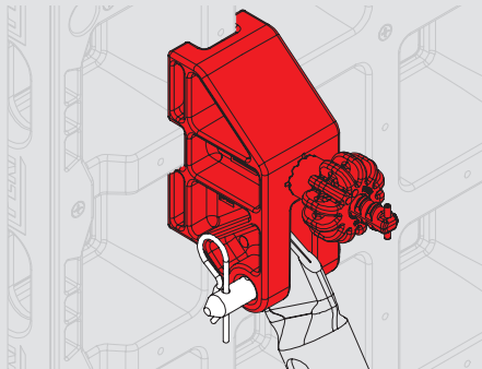
브레이스 커넥터를 사용한 푸쉬-풀 프롭 설치
