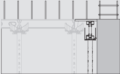
벽체의 앞면에는 VT 20 또는 GT 24 거푸집 거더를 사용하여 필러용 합판을 지지한다. 안정적으로 고정시키기 위해 합판은 못으로 고정한다.
