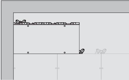
판넬을 위로 올리기 전에 2개의 듀오 커넥터를 사용, 필러 지지대를 판넬의 장변 쪽에 고정한다.
